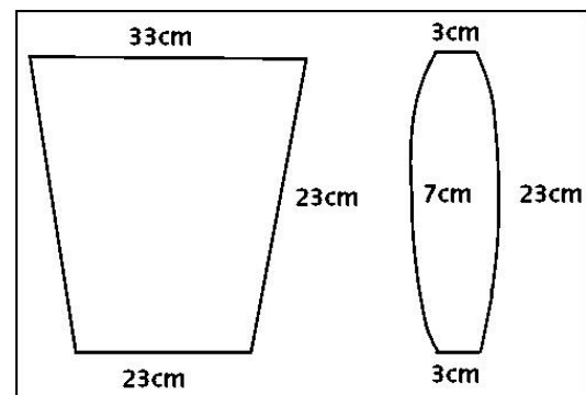
Dimensions des pièces du sac
